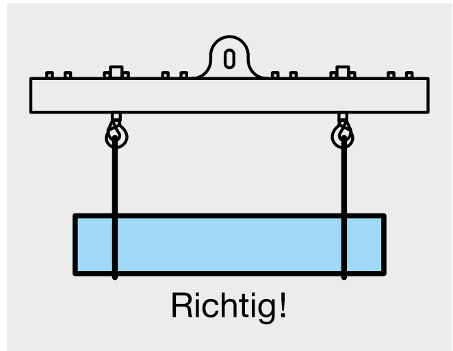
Bild 15-3: Richtiges Anschlagen
